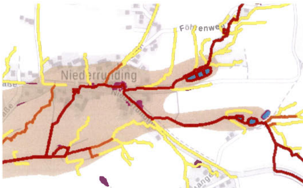
Abb.: wassersensibler Bereich (rosa), potentielle Fließwege bei Starkregen (gelb - mäßiger Abfluss, orange - erhöhter Abfluss, rot - starker Abfluss)
